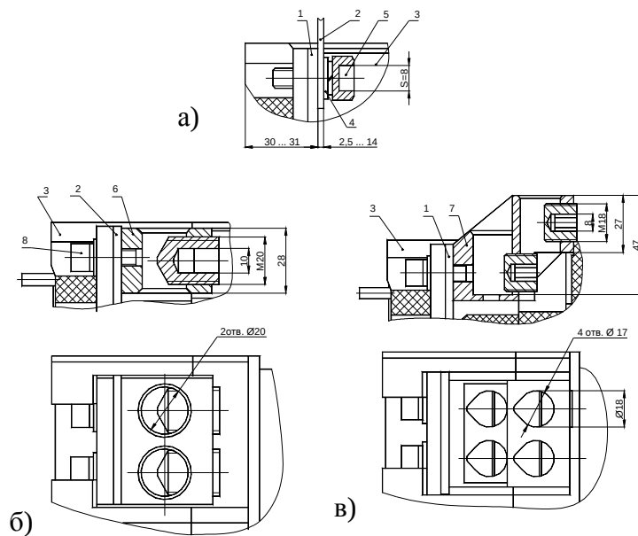
Рисунок 3 - Способы присоединения внешних проводников главной цепи выключателя. а) присоединение шинами или жилами кабеля с кабельным наконечником, б) присоединение двумя кабелями сечением 185 мм 2 без кабельного наконечника, в) присоединение четырьмя кабелями сечением 120 мм 2 без кабельного наконечника. 1- вывод выключателя, 2- шина, 3- выключатель, 4- шайбы, 5- винт М10х25 ГОСТ 11738, 6- двухгнездный зажим, 7- четырехгнездный зажим, 8- болт М8.
