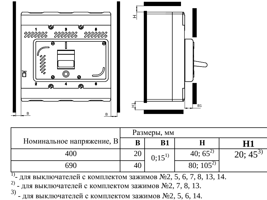
Рисунок 9 - Минимально-допустимые расстояния от выключателей до металлических частей
