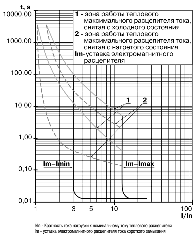
Рисунок F.2 - Время-токовые характеристики выключателей с тепловыми и электромагнитными максимальными расцепителями тока на 16 А; 20 А; 25 А; 31,5 А; 40 А; 50 А
