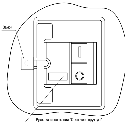
Рисунок С.3 - Запирающее устройство положения "Отключено" выключателей стационарного исполнения
