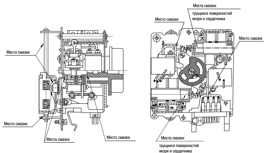
Рисунок В.13 - Места смазки электромагнитного привода
