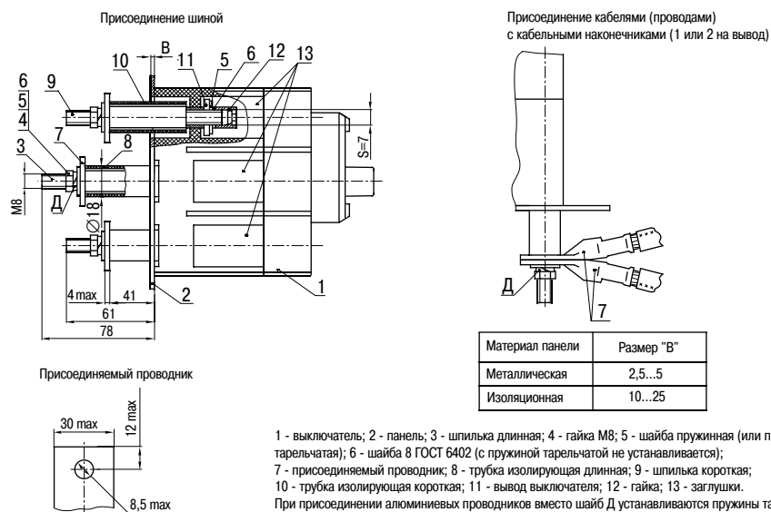
Рисунок D.2 - Способы присоединения внешних проводников к выключателю с задней стороны
