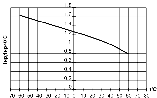
Рисунок F.1 - Зависимость номинального тока выключателя (расцепителя), выраженного в кратностях к номинальному току при 40^\circ C , от температуры окружающего воздуха
