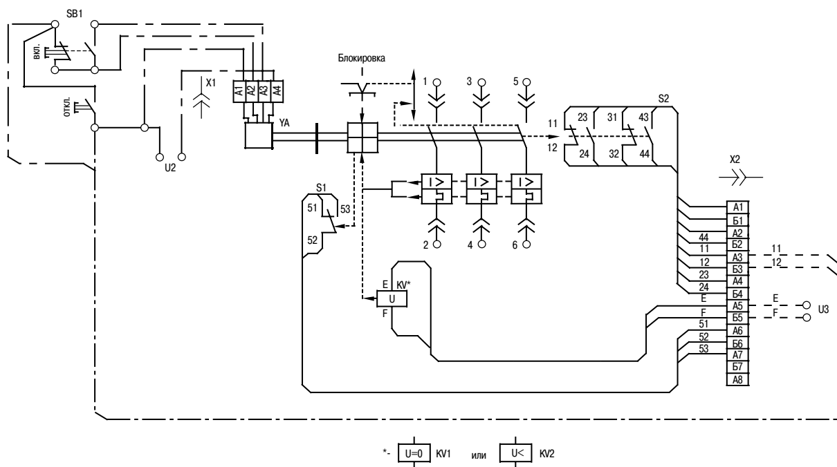
Рисунок Е.10 - Схема электрическая принципиальная выключателей выдвижного исполнения с электромагнитным приводом, с нулевым или минимальным расцепителем напряжения, вспомогательными контактами сигнализации автоматического отключения и свободными контактами
