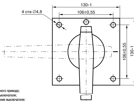
Рисунок В.4 - Выключатель выдвижного исполнения с ручным дистанционным приводом
