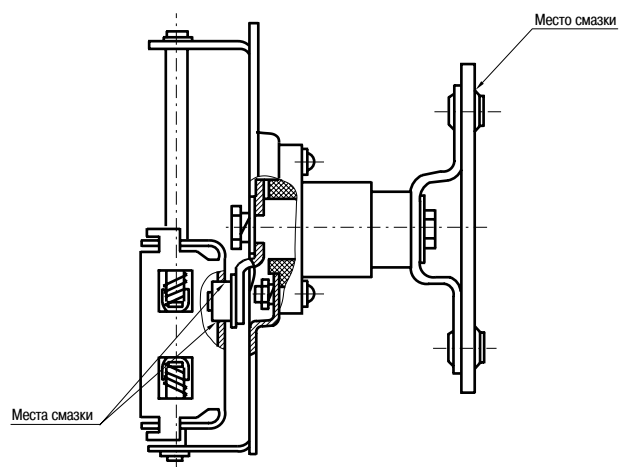
Рисунок В.16 - Места смазки ручного дистанционного привода выключателей выдвижного исполнения
