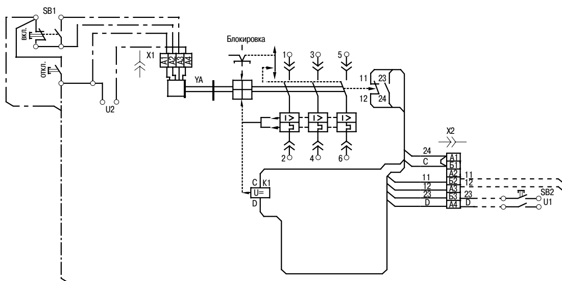
Рисунок Е.4 - Схема электрическая принципиальная выключателей выдвижного исполнения с электромагнитным приводом и независимым расцепителем
