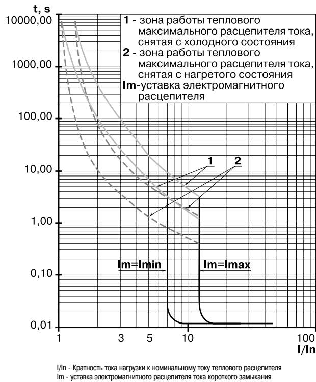
Рисунок F.3 - Время-токовые характеристики выключателей с тепловыми и электромагнитными максимальными расцепителями тока на 63 А; 80 А
