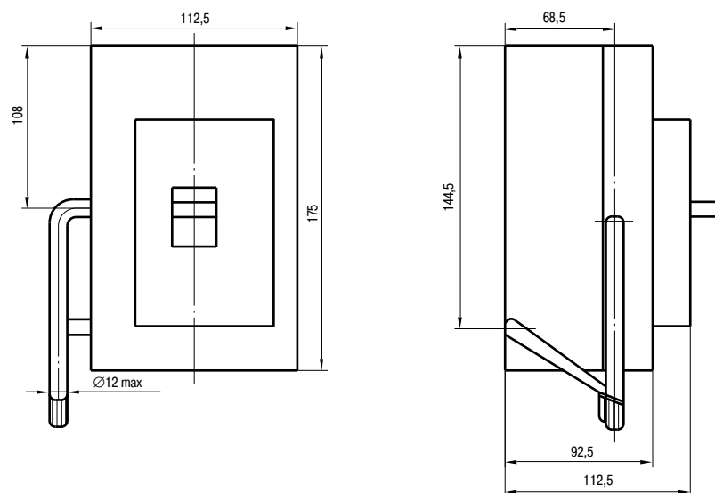
Рисунок В.6 - Расположение выходящих из выключателя проводов от дополнительных сборочных единиц
