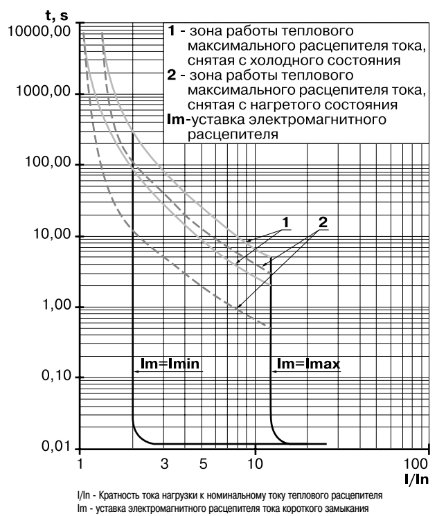
Рисунок F.5 - Время-токовые характеристики выключателей с тепловыми и электромагнитными максимальными расцепителями тока на 160 А; 200 А; 250 А
