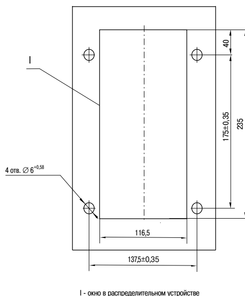
Рисунок В.11 - Отверстия в распределительном устройстве для установки выключателей выдвижного исполнения
