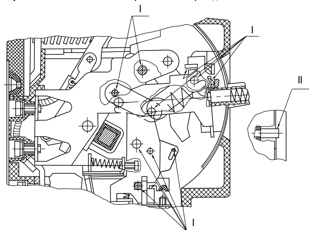
Рисунок В.13 - Места смазки электромагнитного привода
