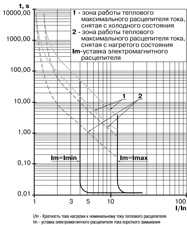
Рисунок F.4 - Время-токовые характеристики выключателей с тепловыми и электромагнитными максимальными расцепителями тока на 100 А; 125 А
