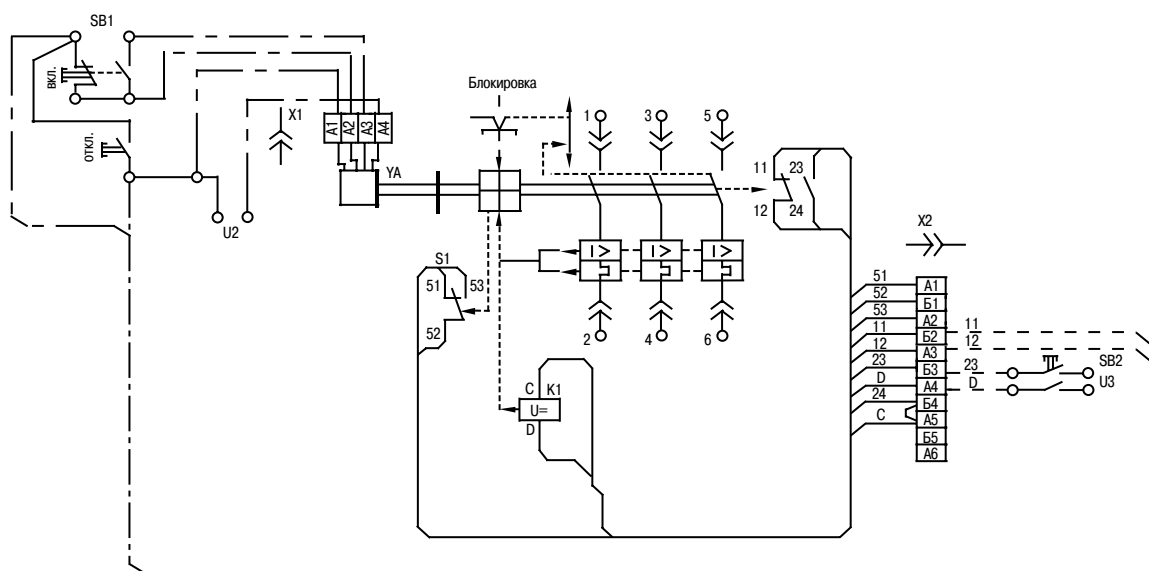
Рисунок Е.10 - Схема электрическая принципиальная выключателей выдвижного исполнения с электромагнитным приводом, с нулевым или минимальным расцепителем напряжения, вспомогательными контактами сигнализации автоматического отключения и свободными контактами
